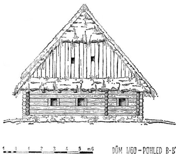
71c. Pfaffenschlag. Rekonstrukce domu I/60
