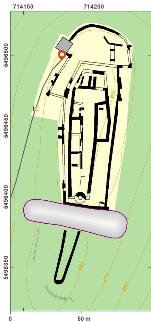
Site plan.
