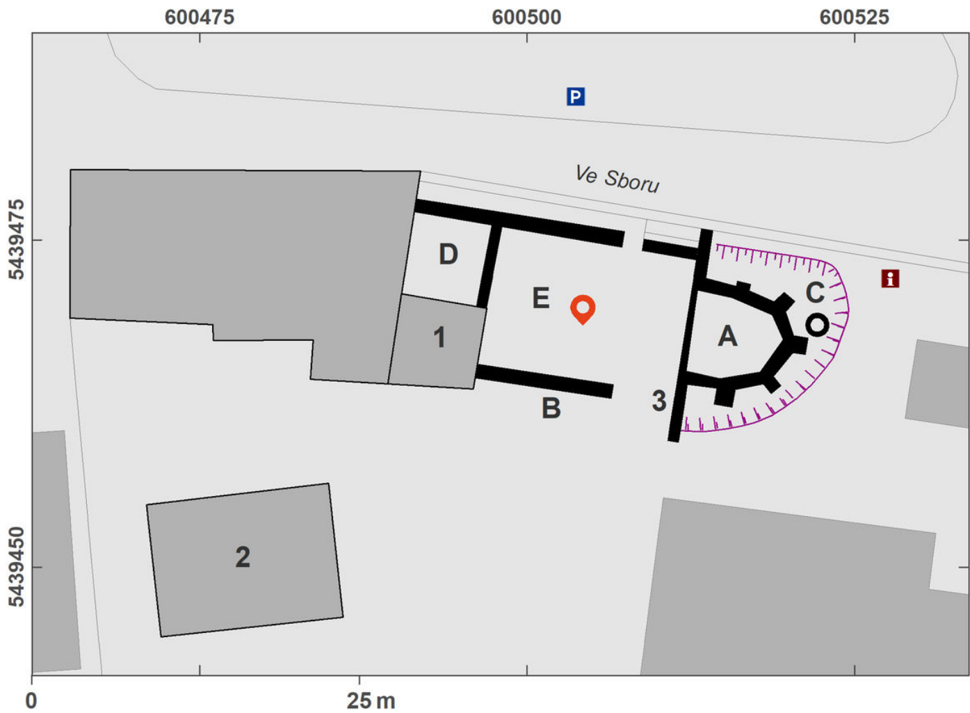
Site plan.
