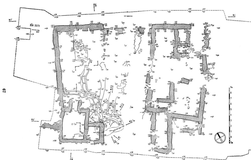
62a. Pfaffenschlag. Púdorys domů IX a X
