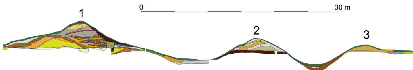
Řez trojitou linií opevnění.
